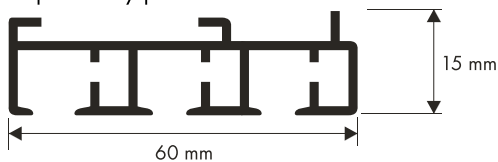
trojdrážkový profil
