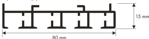
čtyřdrážkový profil
