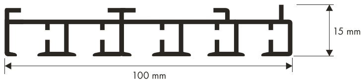
pětidrážkový profil
