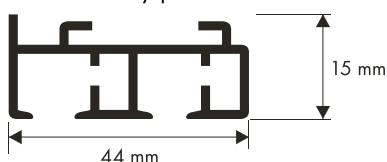
dvoudrážkový profil
